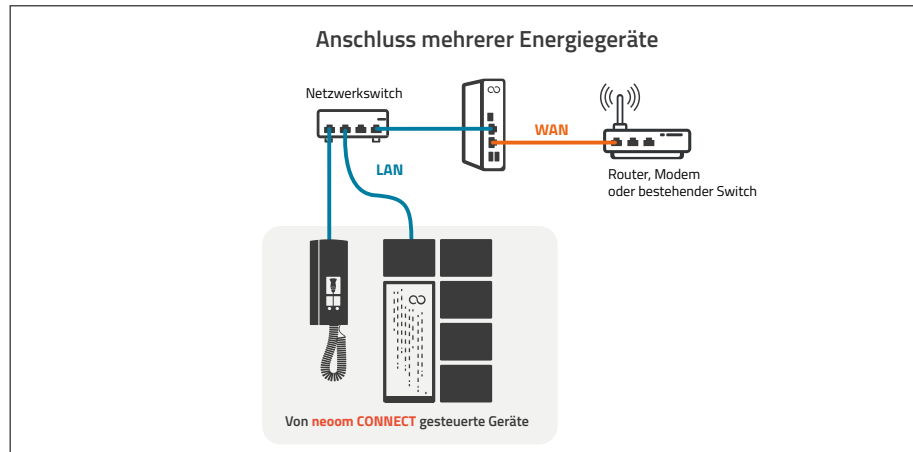
Abbildung2 : Mehrere Energiegeräte werden von neoom Ai gesteuert
