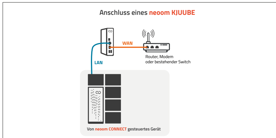
Abbildung 1: nur ein KJUUBE wird von neoom Ai gesteuert
